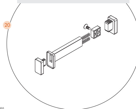
Detalle kit muelle presión instalación dentro marco
